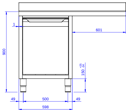
Oldalnézet
